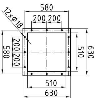
Příruba P1
